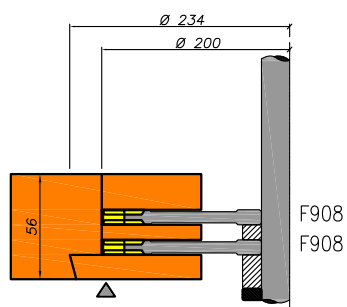
Waterslag dorpelsponning
