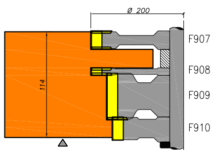
Onderdorpel
