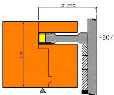
Ramen 56 mm
